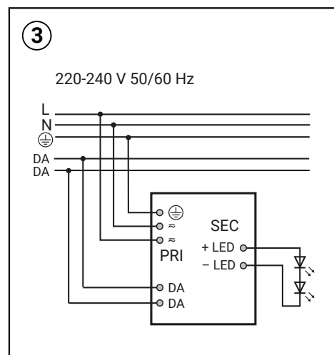
DALI DIM
